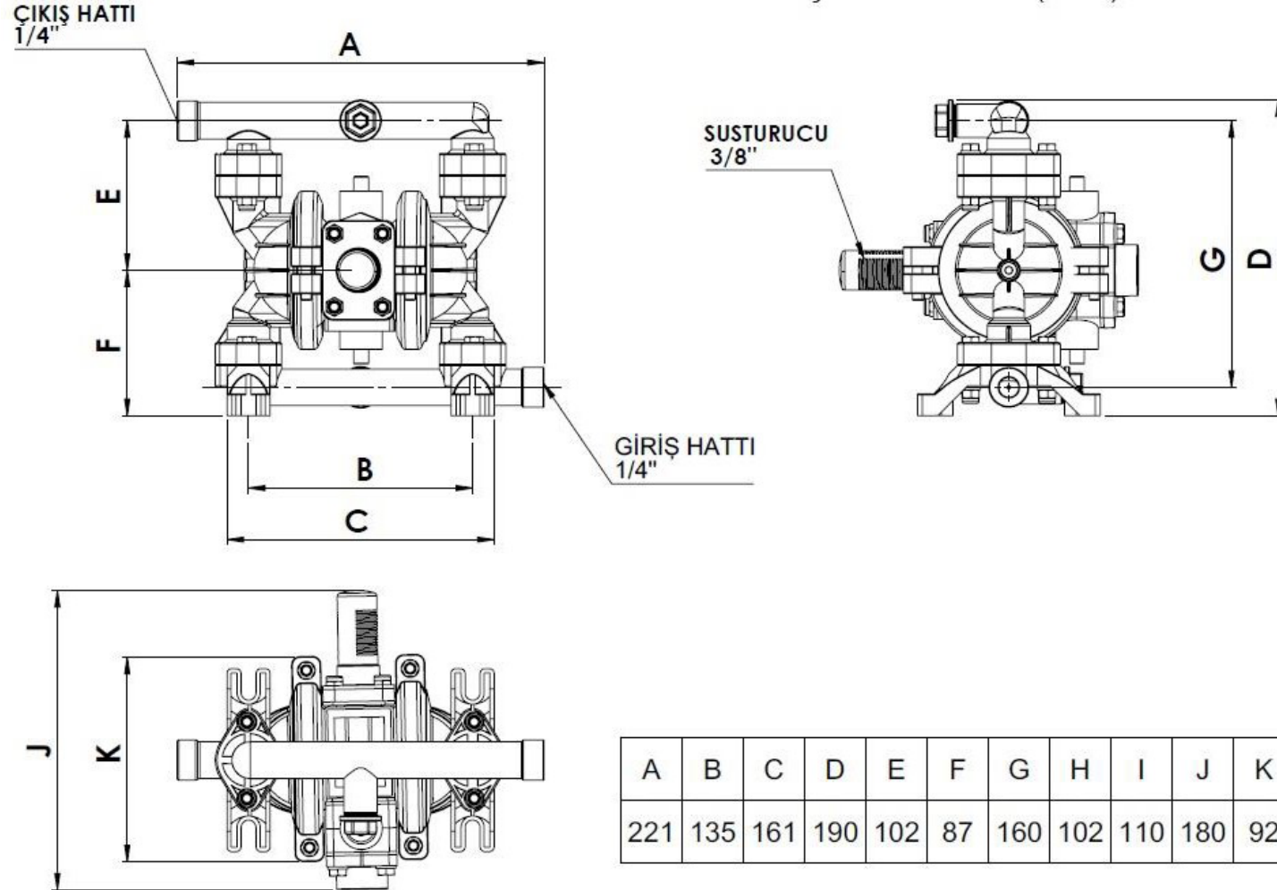
DP 03 PLASTİK POMPA METRİK ÖLÇÜLENDİRME (mm.)
